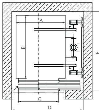
przekrój poziomy szybu 2 drzwi
