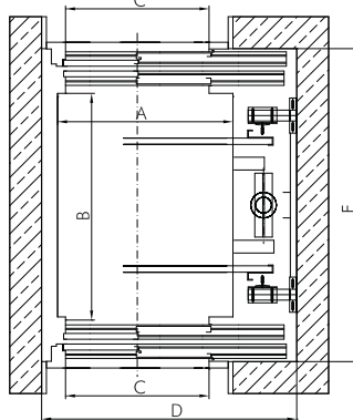
przekrój poziomy szybu 2 drzwi
