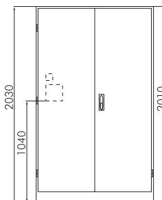
maszynownia prefabrykowana
