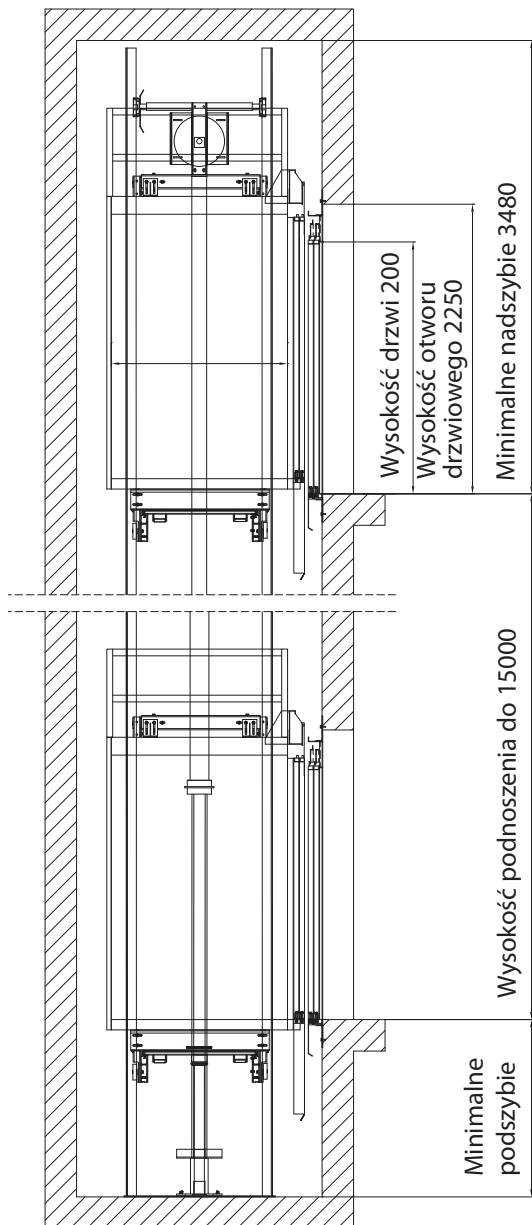
przekrój szybu
